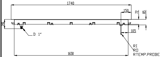
Front aanzicht
