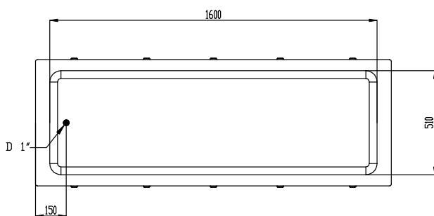
Boven aanzicht
