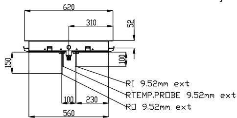
Zij aanzicht
